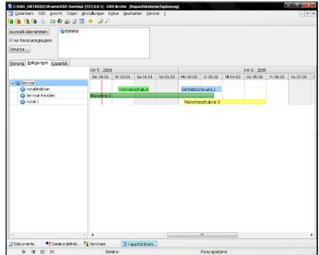
Grafische Kapazitätsplanung
